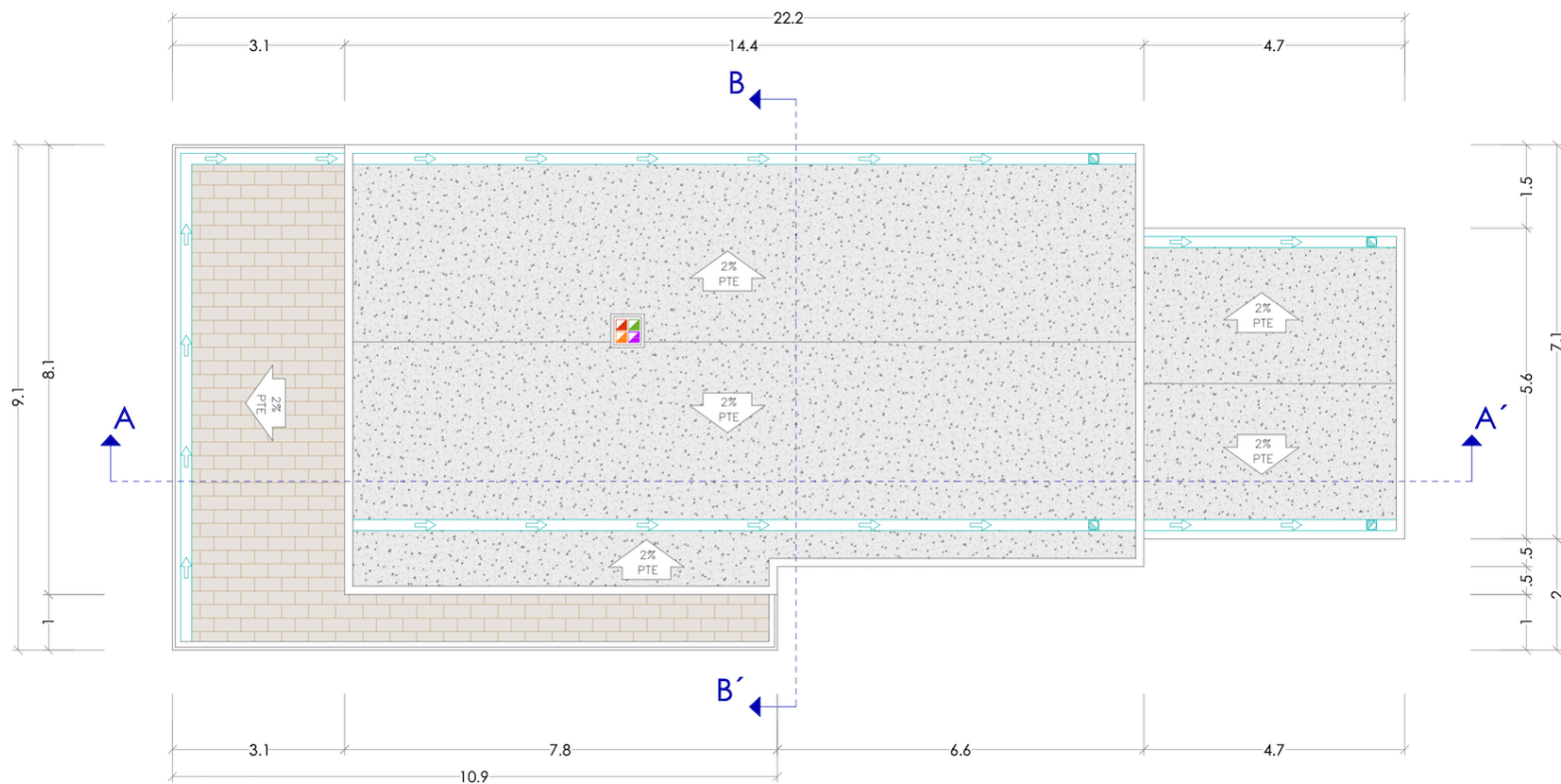
PLANTA DE CUBIERTAS
